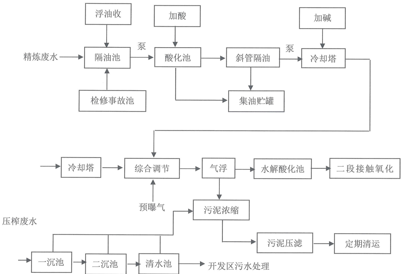
图 1 厂内废水处理工艺流程图
