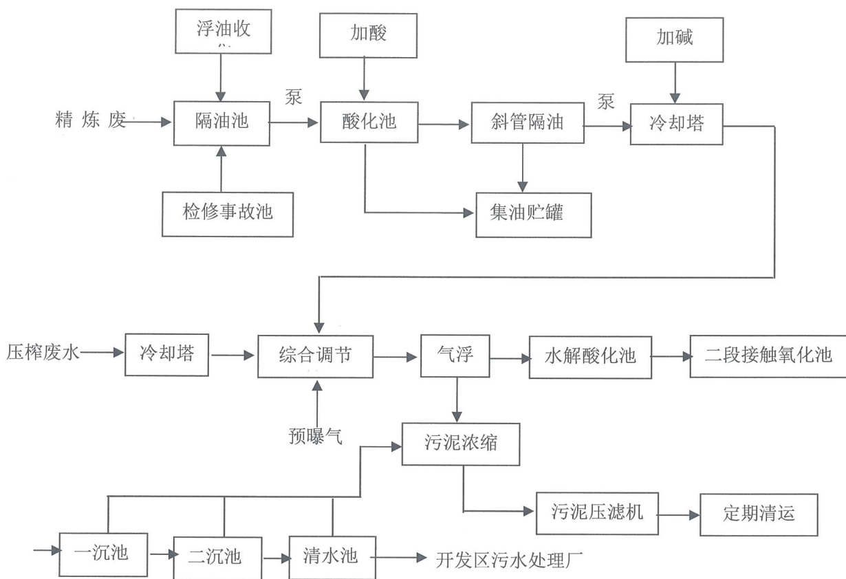
图 4-1 厂内废水处理工艺流程图
